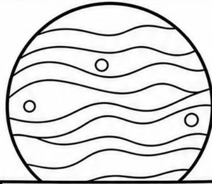
VENUS
