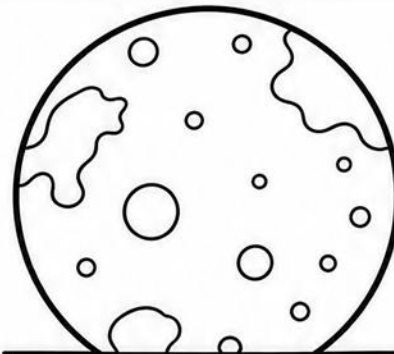
MARS
