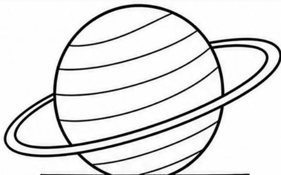
URANUS
