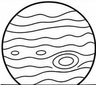
JUPITER
