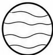
VENUS
