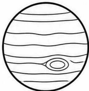
JUPITER
