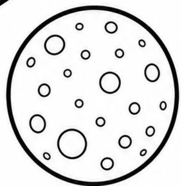
CALLISTO
