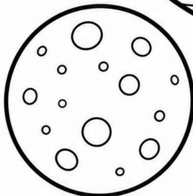
GANYMEDE
